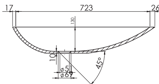
SECCIÓN A-A
