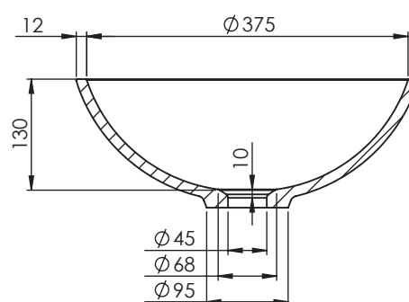
SECCIÓN A-A
