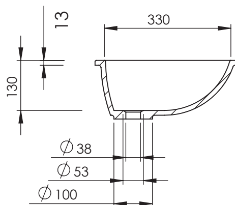
SECCIÓN A-A
