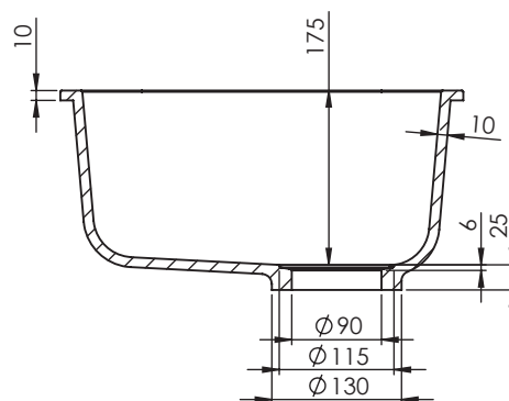
SECCIÓN A-A
