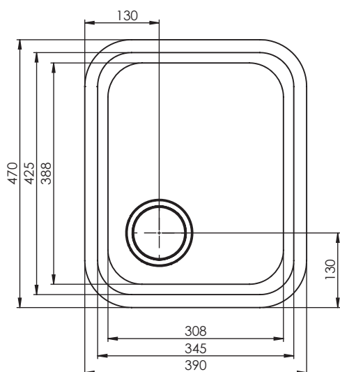
VISTA SUPERIOR
