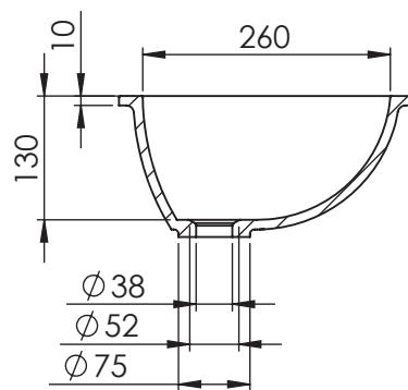
SECCIÓN A-A
