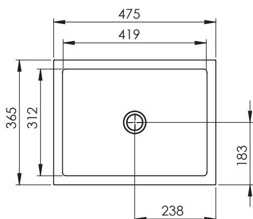
VISTA SUPERIOR
