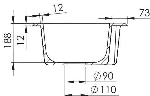
SECCIÓN A-A
