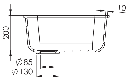
SECCIÓN A-A
