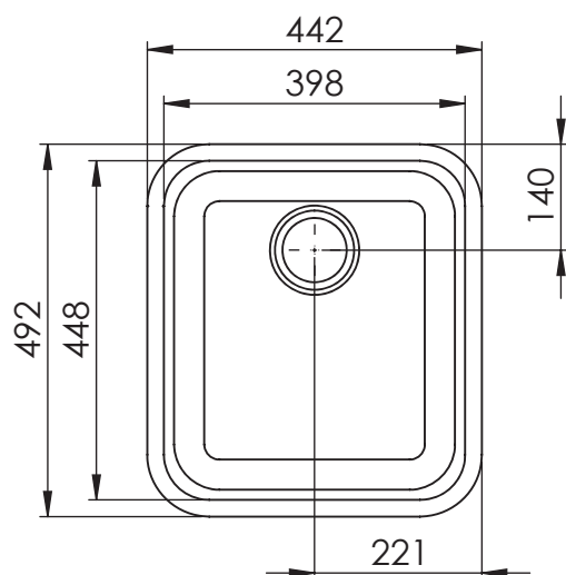
VISTA SUPERIOR
