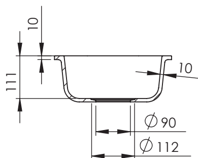
SECCIÓN A-A
