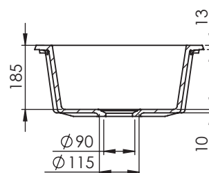
SECCIÓN B-B
