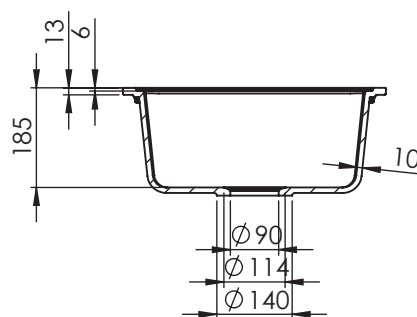
SECCIÓN A-A
