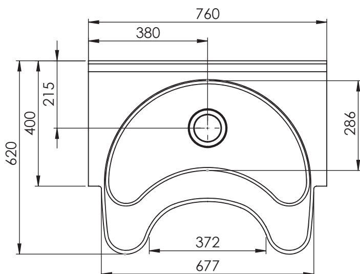
VISTA SUPERIOR
