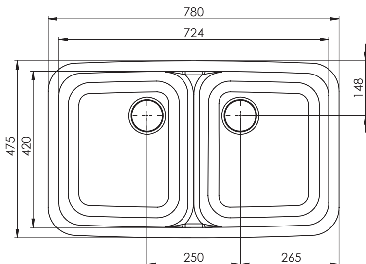
VISTA SUPERIOR
