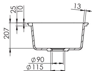
SECCIÓN B-B
