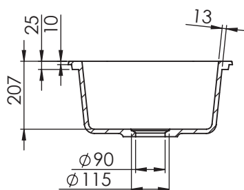
SECCIÓN A-A
