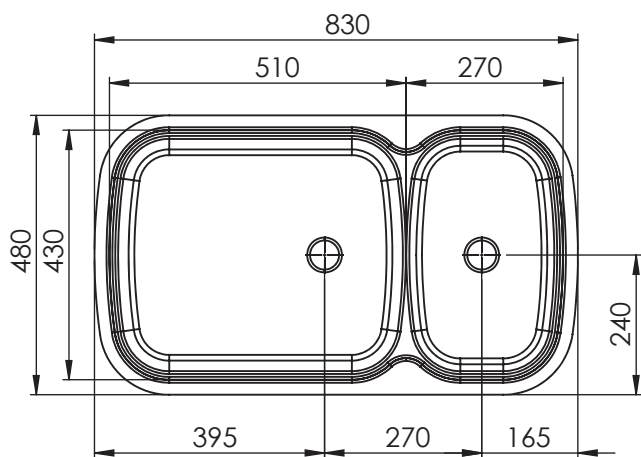
VISTA SUPERIOR
