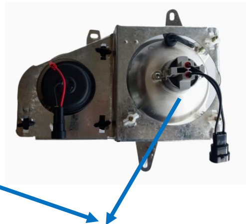
Portalámparas H7 Baja con chicote de conexión
