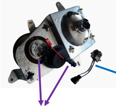
Portalámparas H1 Alta con chicote de conexión
