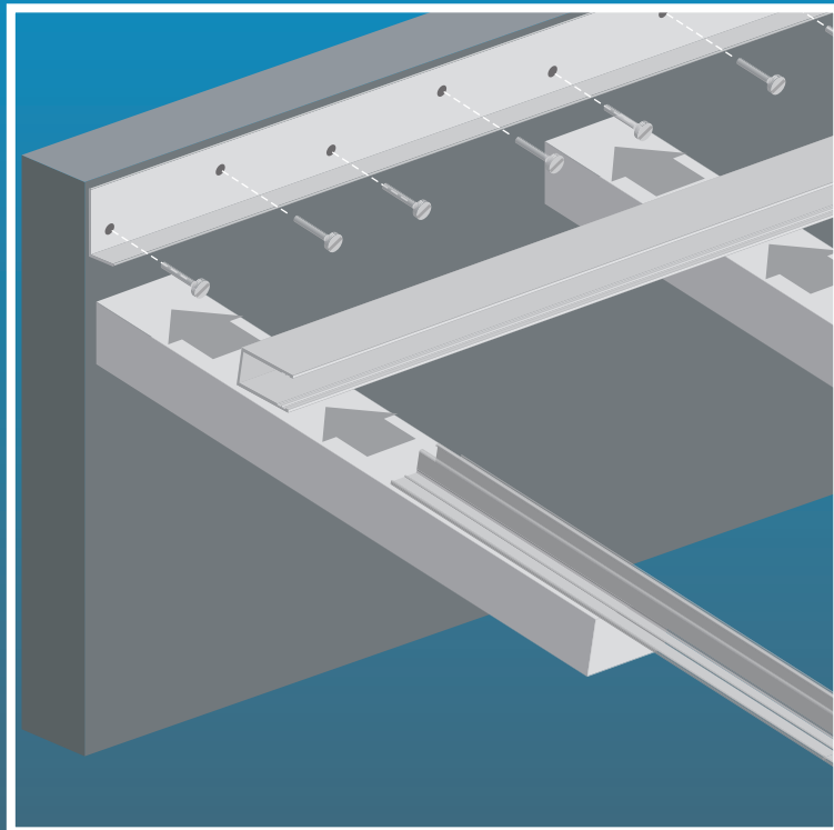
1. Fijación de babetas perimetrales
