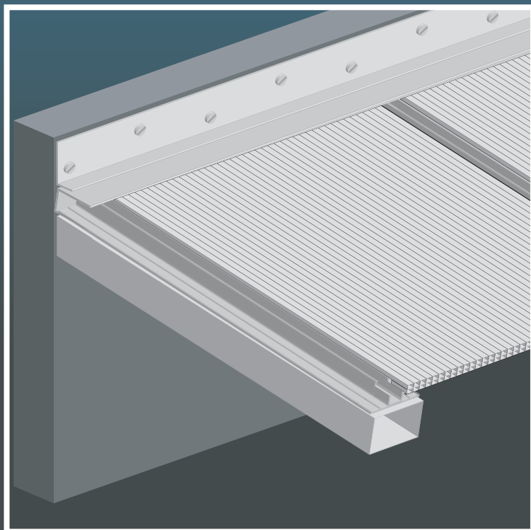
3. Instalación de placas alveolares
