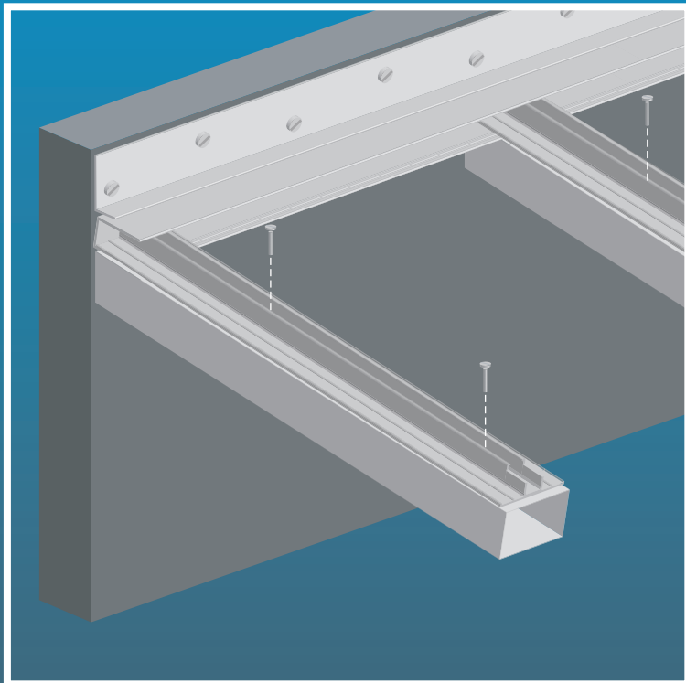
2. Fijación de perfiles superior y MF
