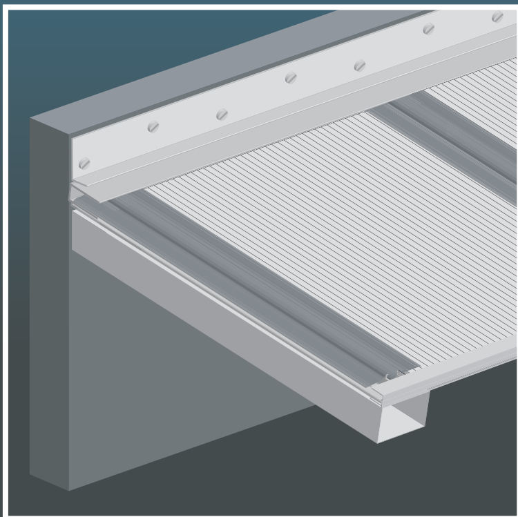
4. Encastre de Goma MF y perfil inferior
