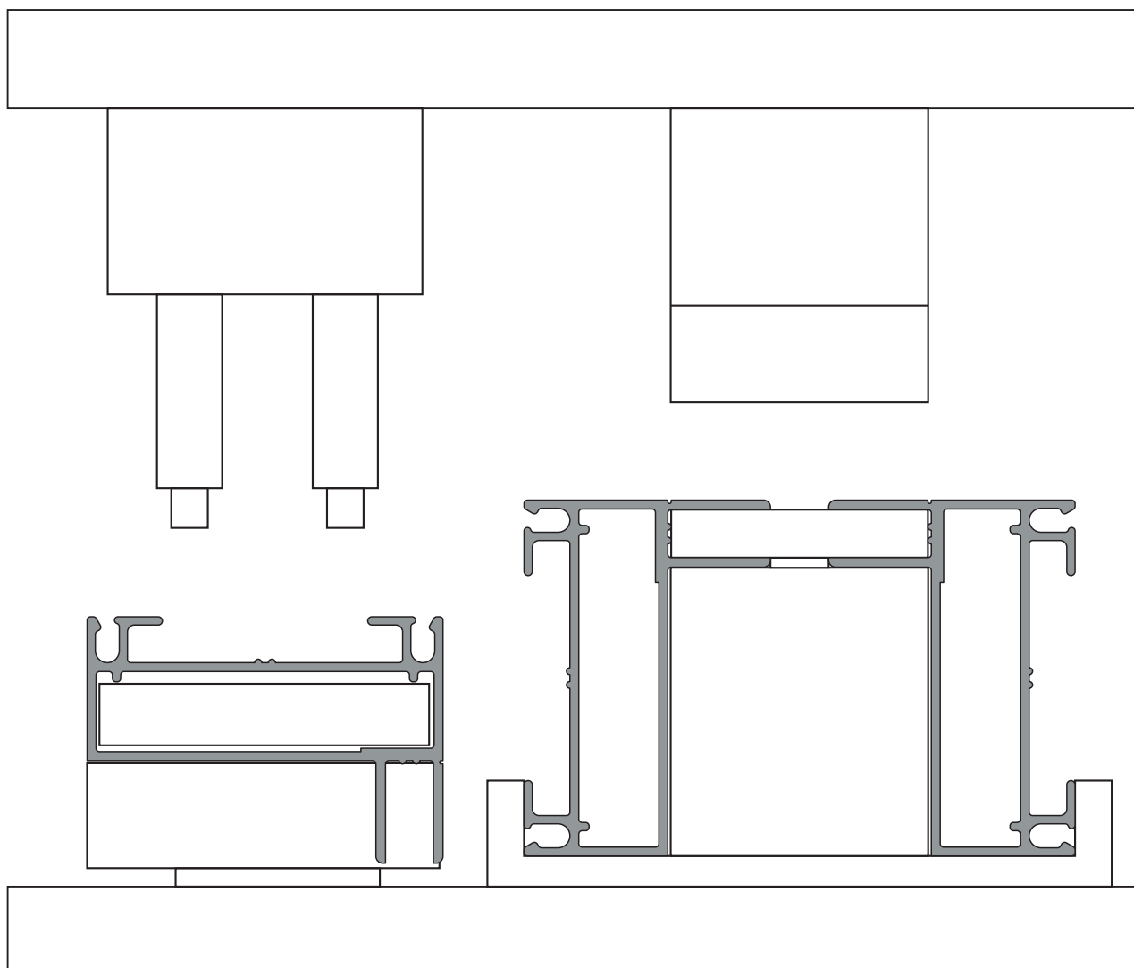
Perforaciones y alobj. de tornillos 7714
