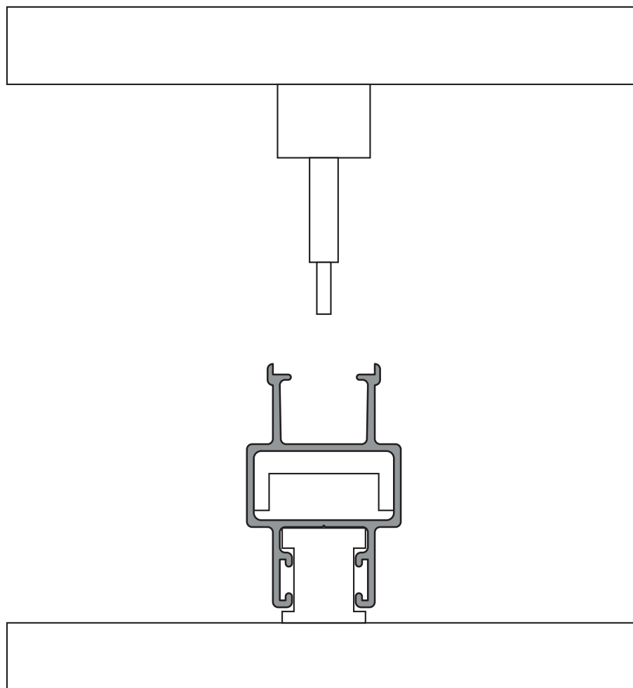
Mecanizado de parante lateral y central 3 / 4
