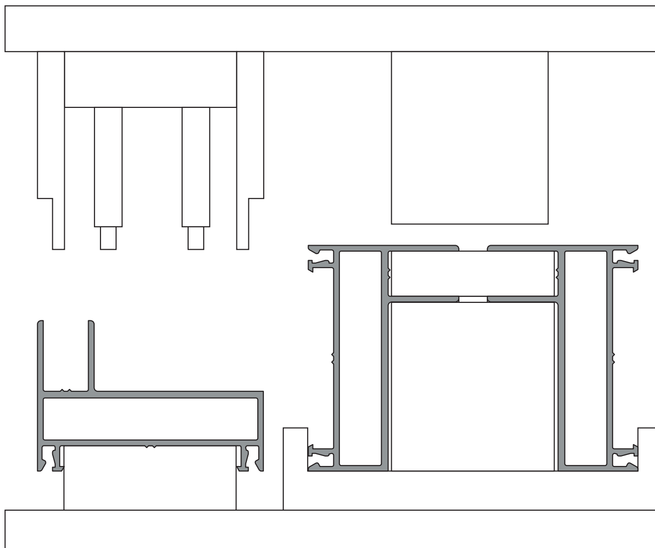
Mecanizado jambas de marco para encastre de umbral y dintel 6036
