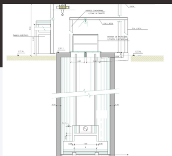
Nuevo Sistema de Desagües Cloacales para la localidad de Laguna Blanca. Formosa.
