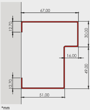
Detalle marco ROMEX
