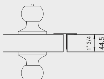
Detalle Perfil Cubrejunta
