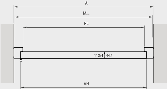
Sección horizontal
